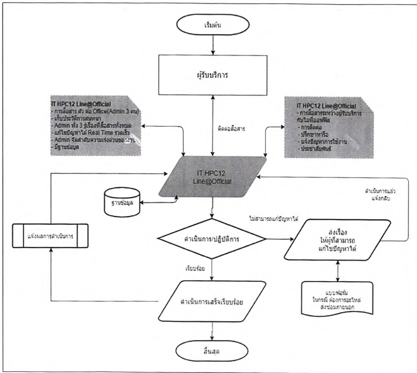
ผัง FlowChart พัฒนาระบบ สารสนเทศ IT HPC12 Line@Official ของศูนย์อนามัยที่ 12 ยะลา
